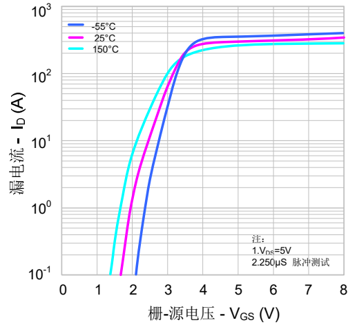
图 2. 传输特性
